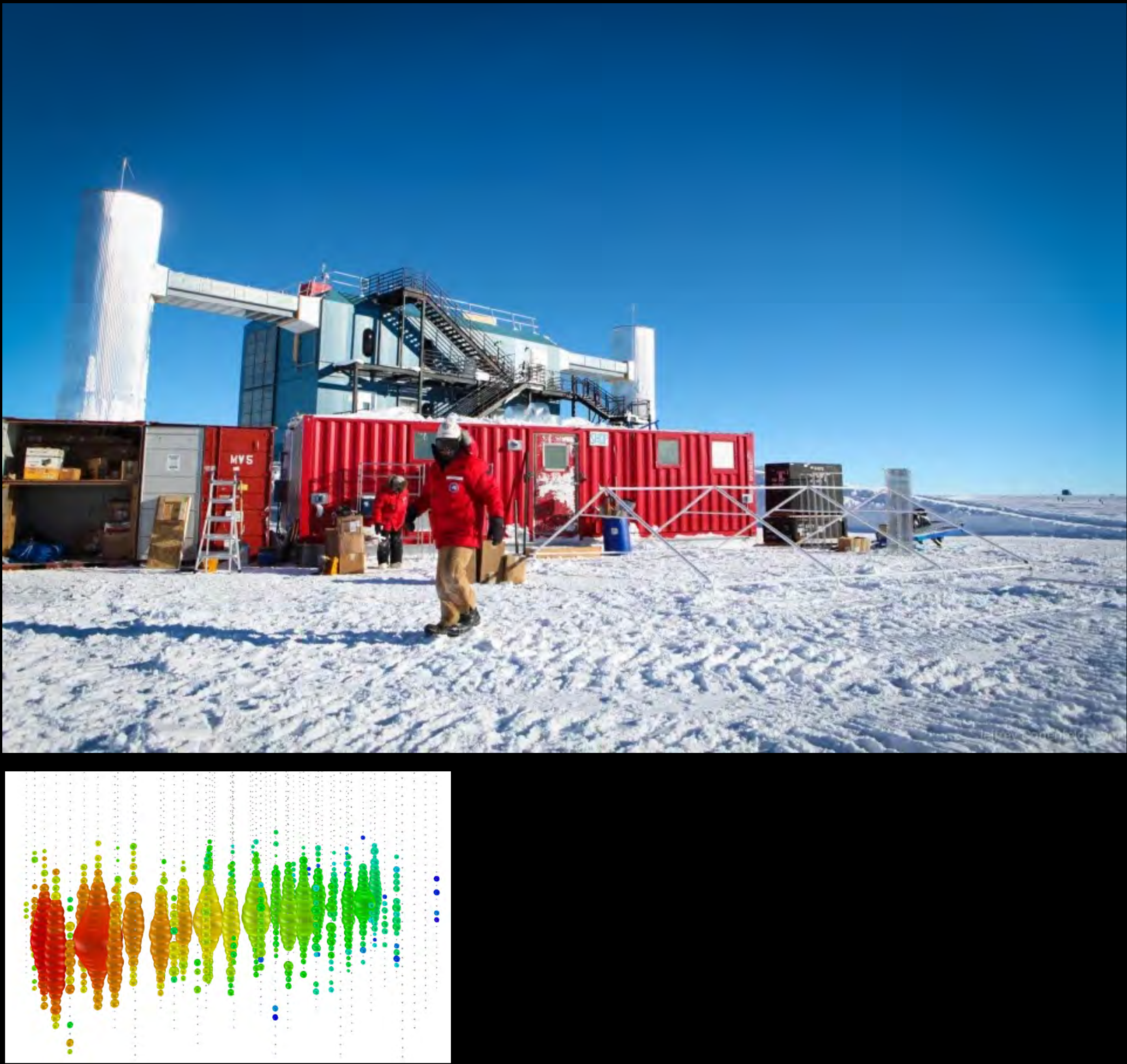
IceCube Neutrino Observatorium am Südpol: 1 km 3 Volumen
